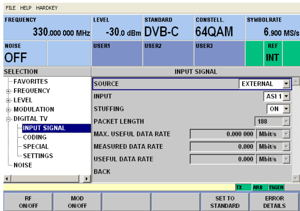
Fig. 6-1: DIGITAL TV menu
